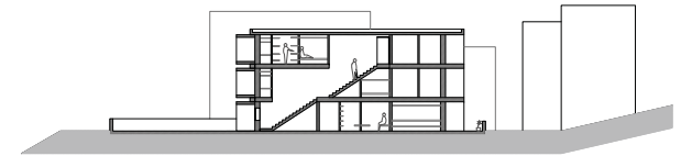
schnitt cc
