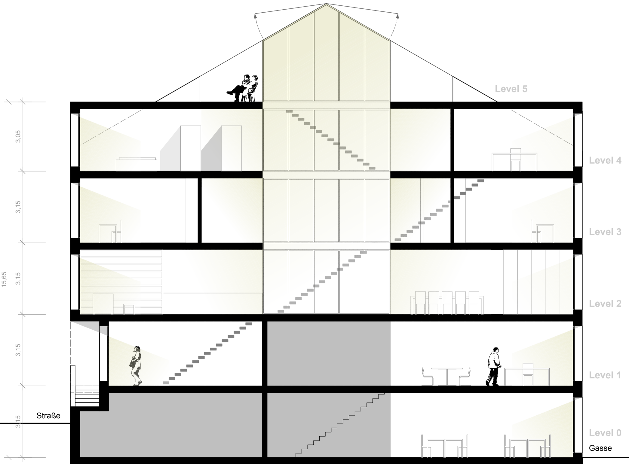
Schnitt A-A
