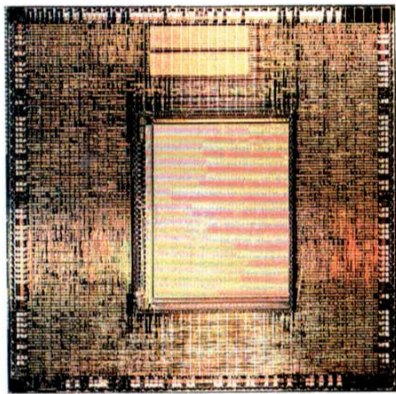
chip zora gesamtbild dimension 12.7mm x 12.7mm
