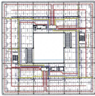
fha windisch hauptgebäude koordinationsplan medienschliessung dimension 52.8m x 52.8m
